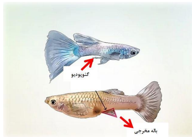
شکل ۶: تعیین جنسیت ماهی گوپی بر اساس باله‌ی مخرجی.
