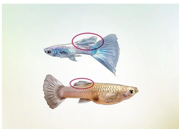
شکل ۴: تشخیص جنسیت ماهی گویی بر اساس باله پستی
