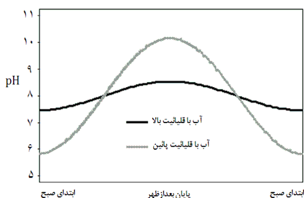
شکل ۳: تغییرات pH در آب‌های با میزان کلیائیت بالا و پائین در طی ۲۴ ساعت (با اندکی تغییر برگرفته از (Wurts and Durborow, 1992)
